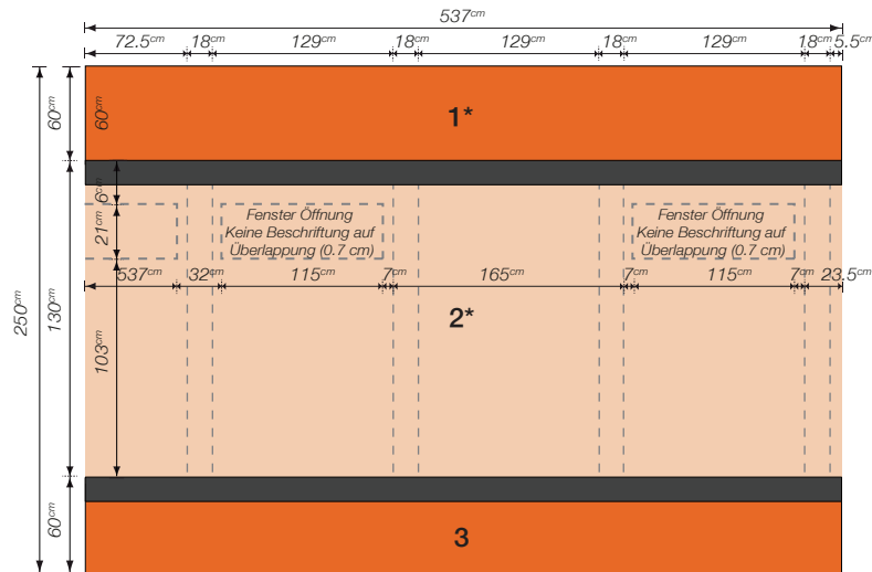
MEGA 12 - Doppelgelenktram Skizze für den Grafiker und den Drucker
